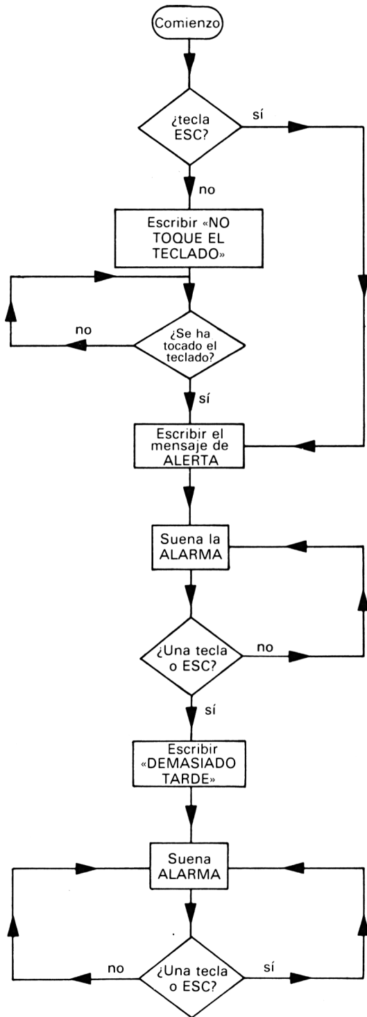
Figura 7.1 Alarma contra intrusos.
